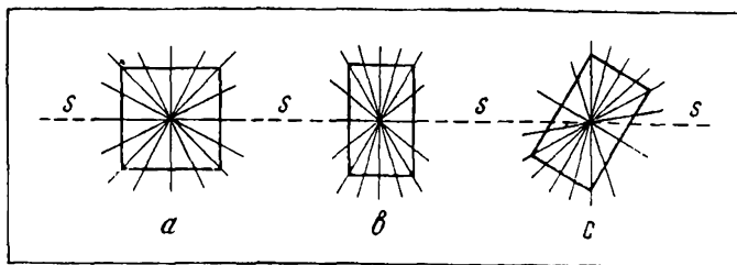
Рис. 1. Элемент объема, показанный символически:
